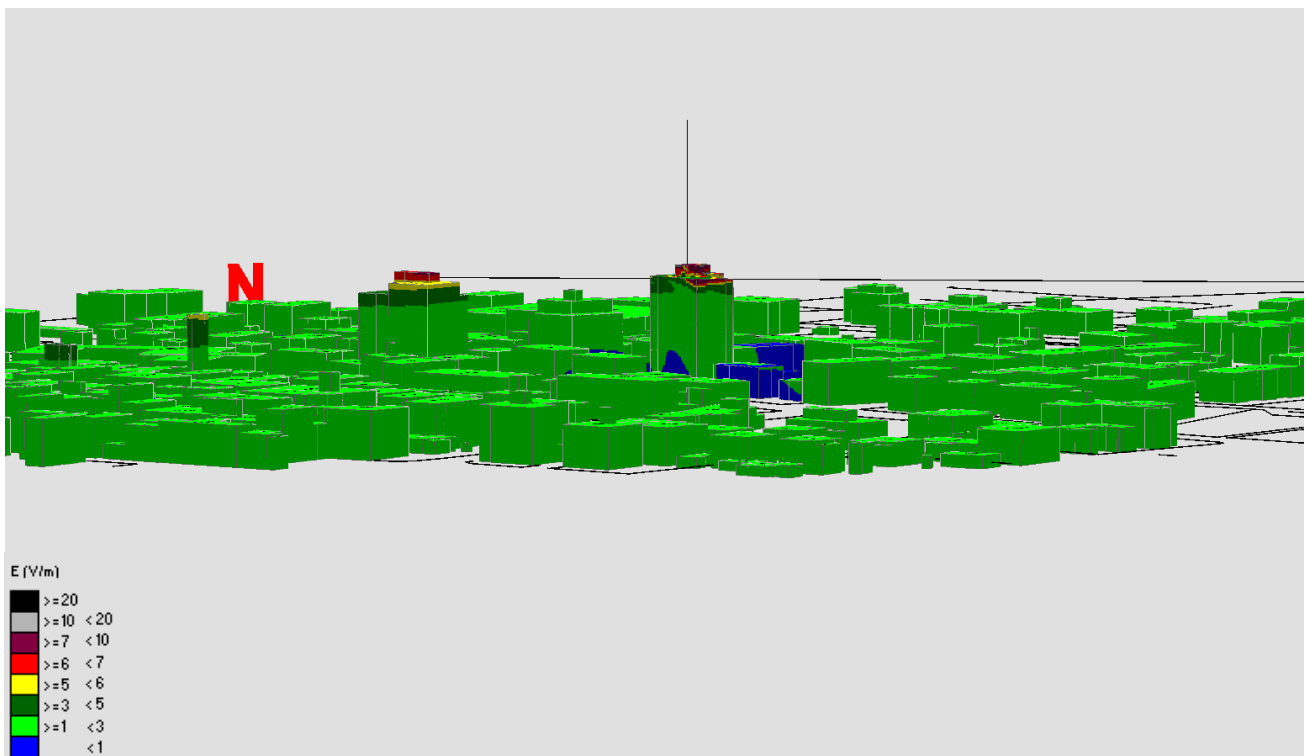
Fig. 30 Impatto elettromagnetico – Zona Castel Franco Centro – Vista Laterale 2
