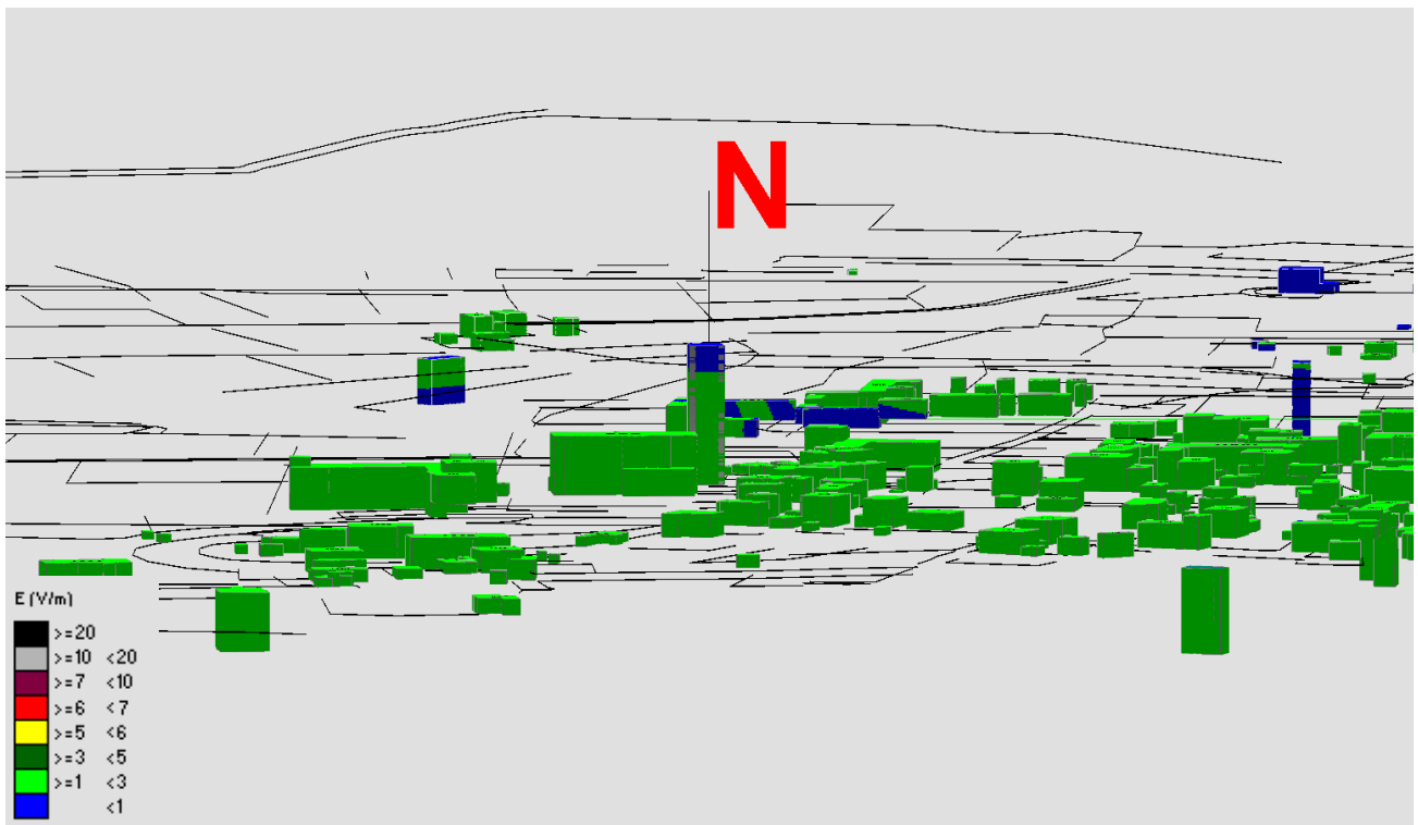
Fig. 5 Impatto elettromagnetico – Zona Cimitero Orentano – Vista Laterale 2
