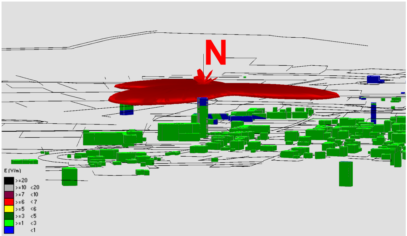
Fig. 4 Impatto elettromagnetico – Zona Cimitero Orentano – Vista Laterale 1
