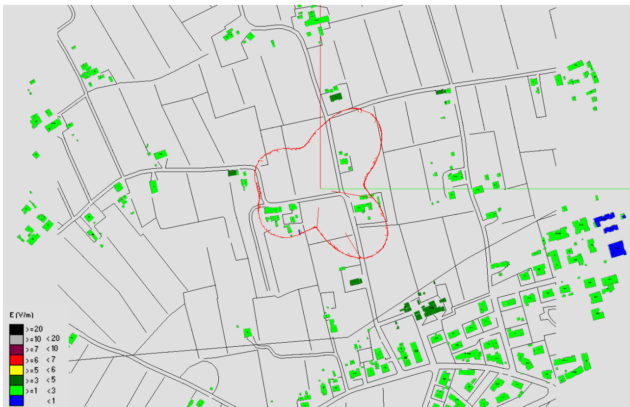
Fig. 18 Impatto elettromagnetico – Zona Castel Franco Via dell'Iserone – Vista dall'alto
