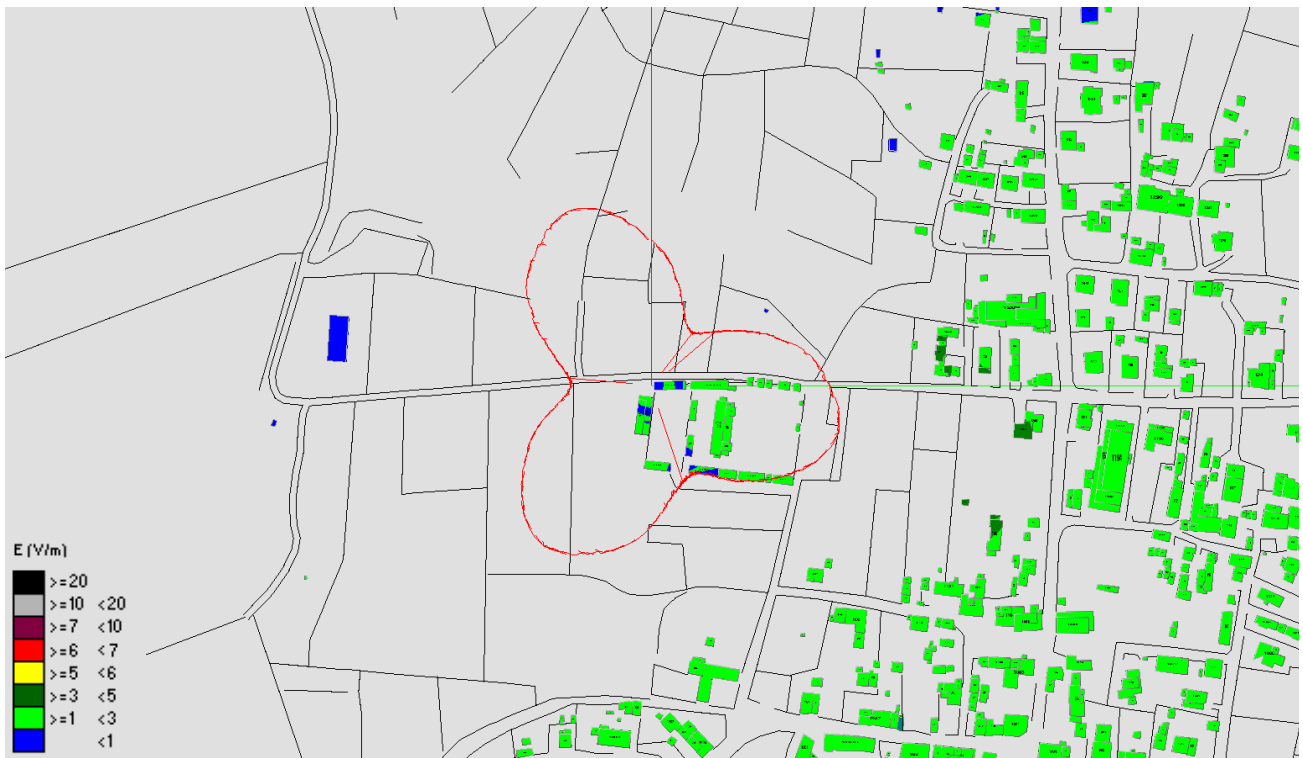
Fig. 3 Impatto elettromagnetico – Zona Cimitero Orentano – Vista dall'alto
