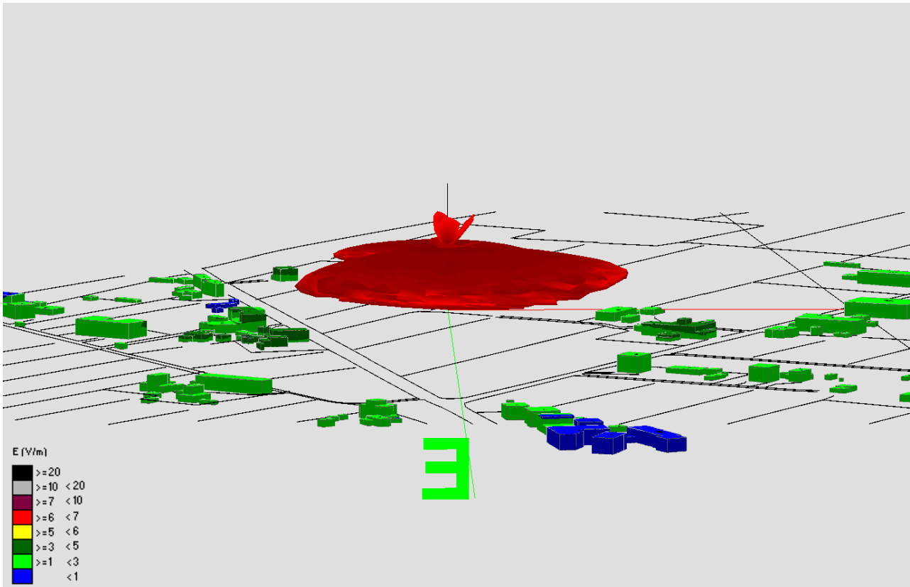
Fig. 24 Impatto elettromagnetico – Zona SP Francesca Sud – Vista Laterale 1
