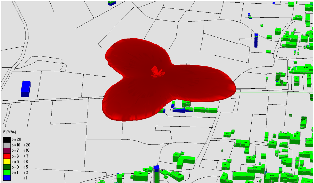
Fig. 2 Impatto elettromagnetico – Zona Cimitero Orentano – 0°/Nord
