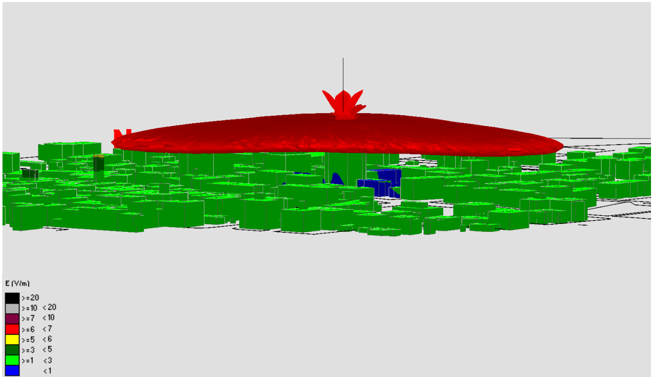
Fig. 29 Impatto elettromagnetico – Zona Castel Franco Centro – Vista Laterale 1
