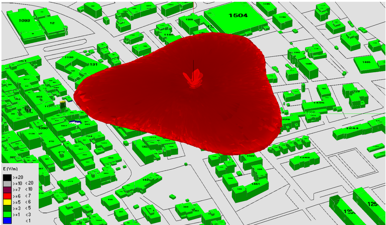
Fig. 27 Impatto elettromagnetico – Zona Castelfranco Centro – 0°/Nord
