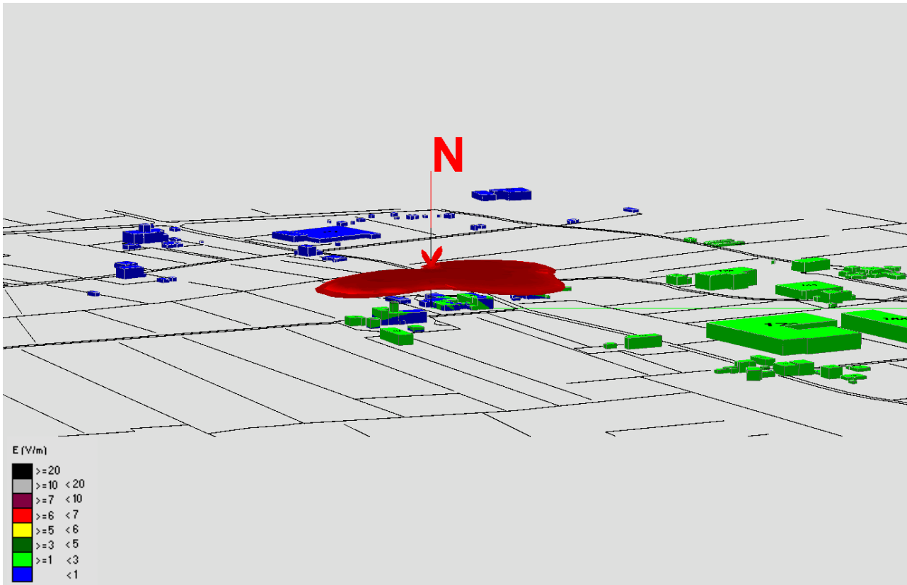
Fig. 14 Impatto elettromagnetico – Zona Via Aiale – Vista Laterale 1
