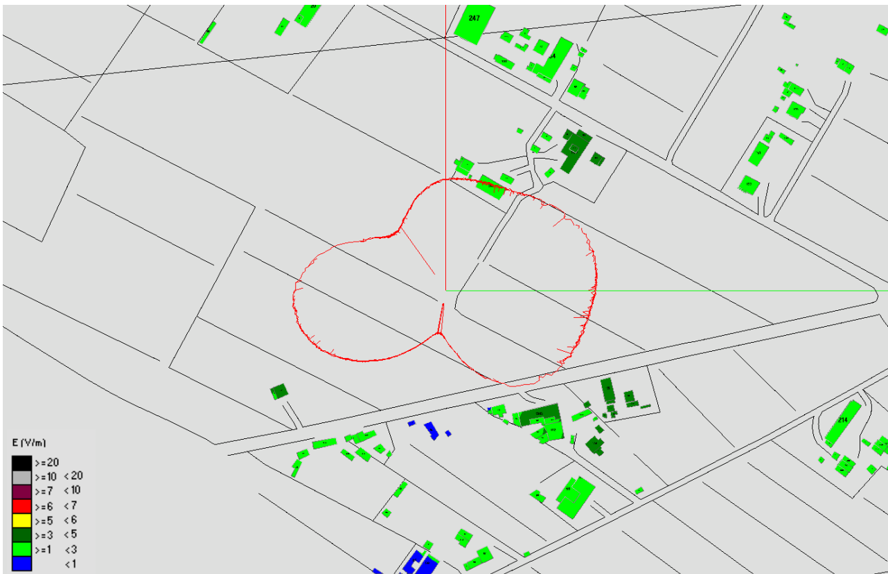
Fig. 23 Impatto elettromagnetico – Zona SP Francesca Sud – Vista dall'alto
