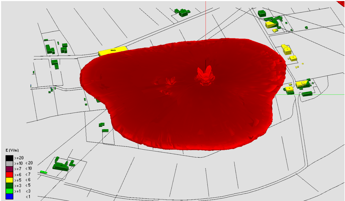
Fig. 32 Impatto elettromagnetico – Zona Via dei Tavi – 0°/Nord
