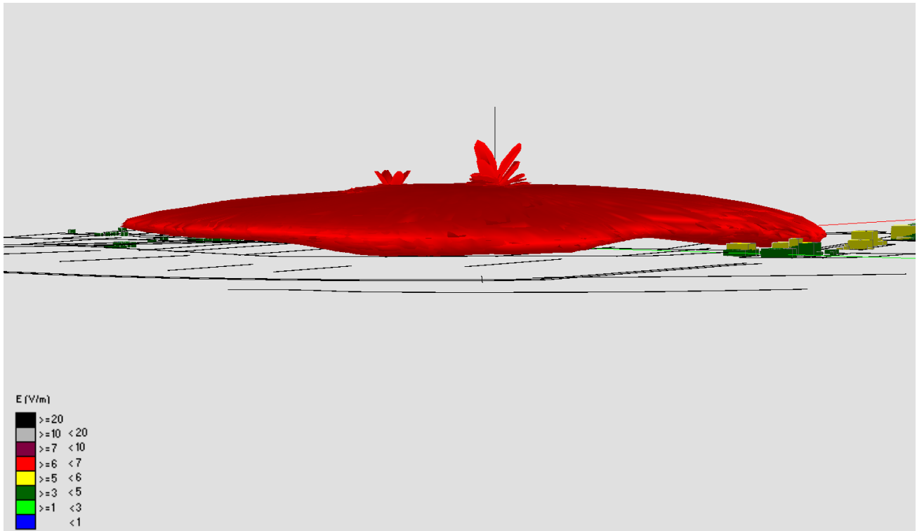
Fig. 34 Impatto elettromagnetico – Zona Via dei Tavi – Vista Laterale 1
