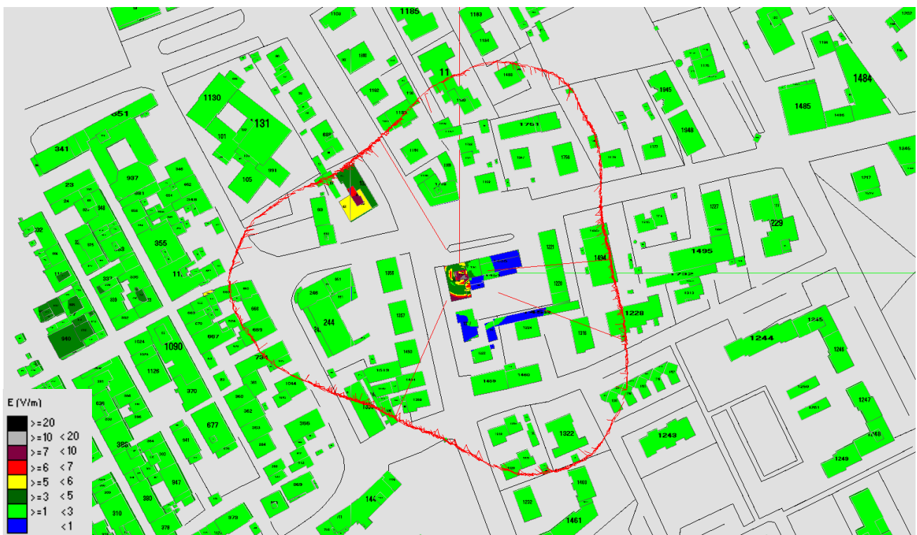
Fig. 28 Impatto elettromagnetico – Zona Castelfranco Centro – Vista dall'alto
