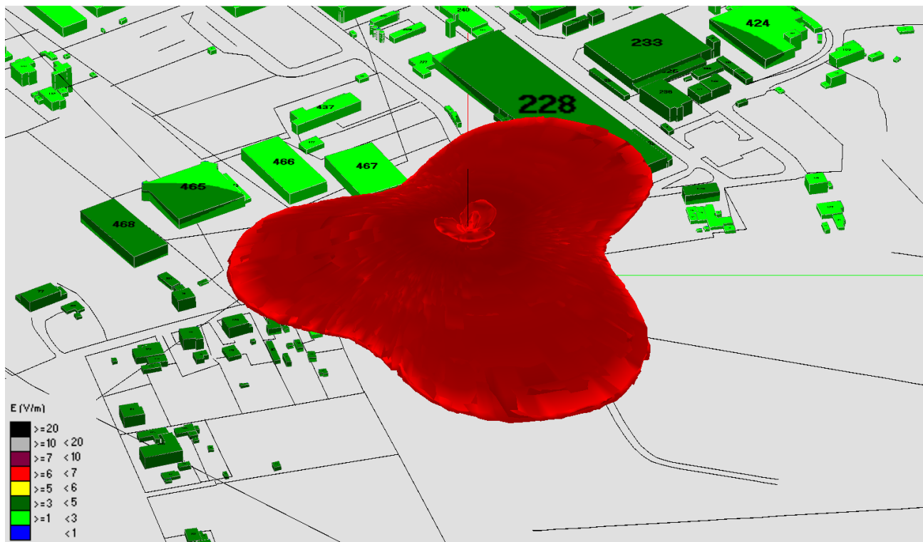
Fig. 37 Impatto elettromagnetico – Zona Via dei Tavi Centrale ENEL – 0°/Nord
