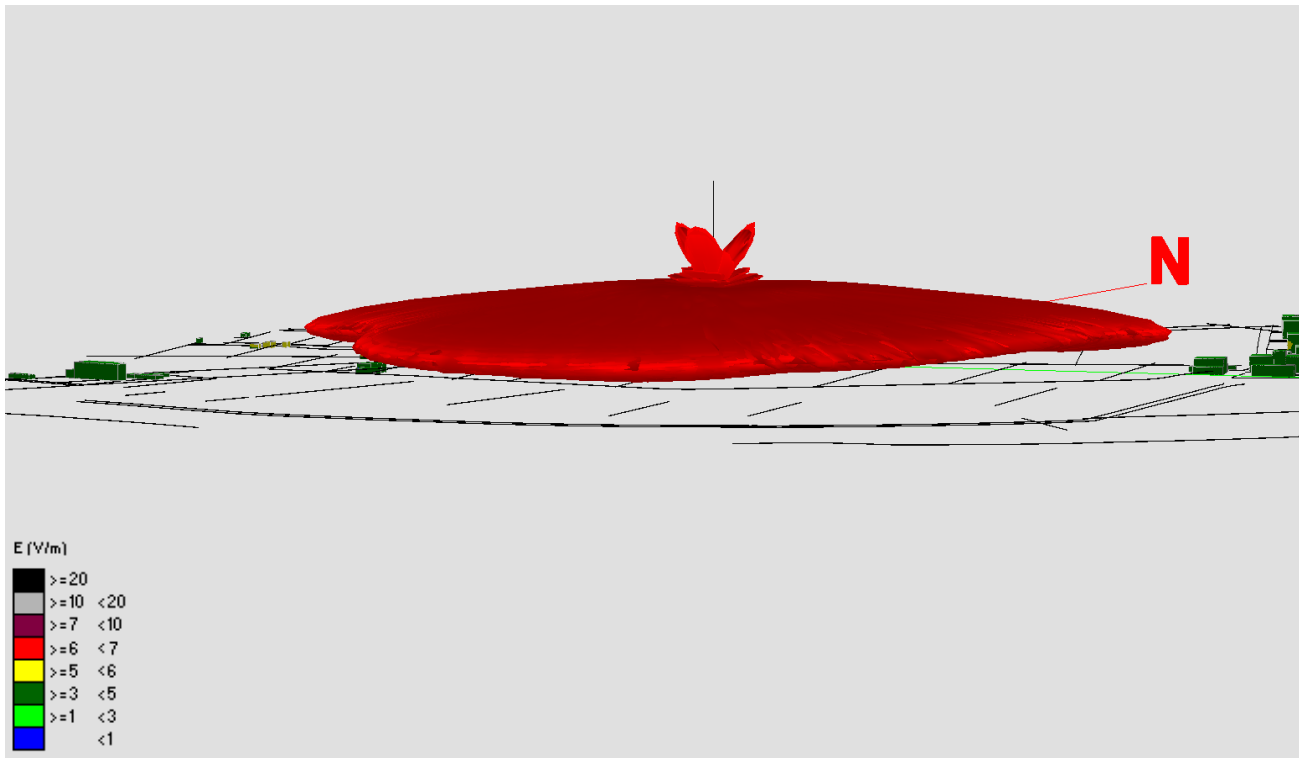
Fig. 29 Impatto elettromagnetico - Zona Area Comunale Via dei Tavi - Vista Laterale 1
