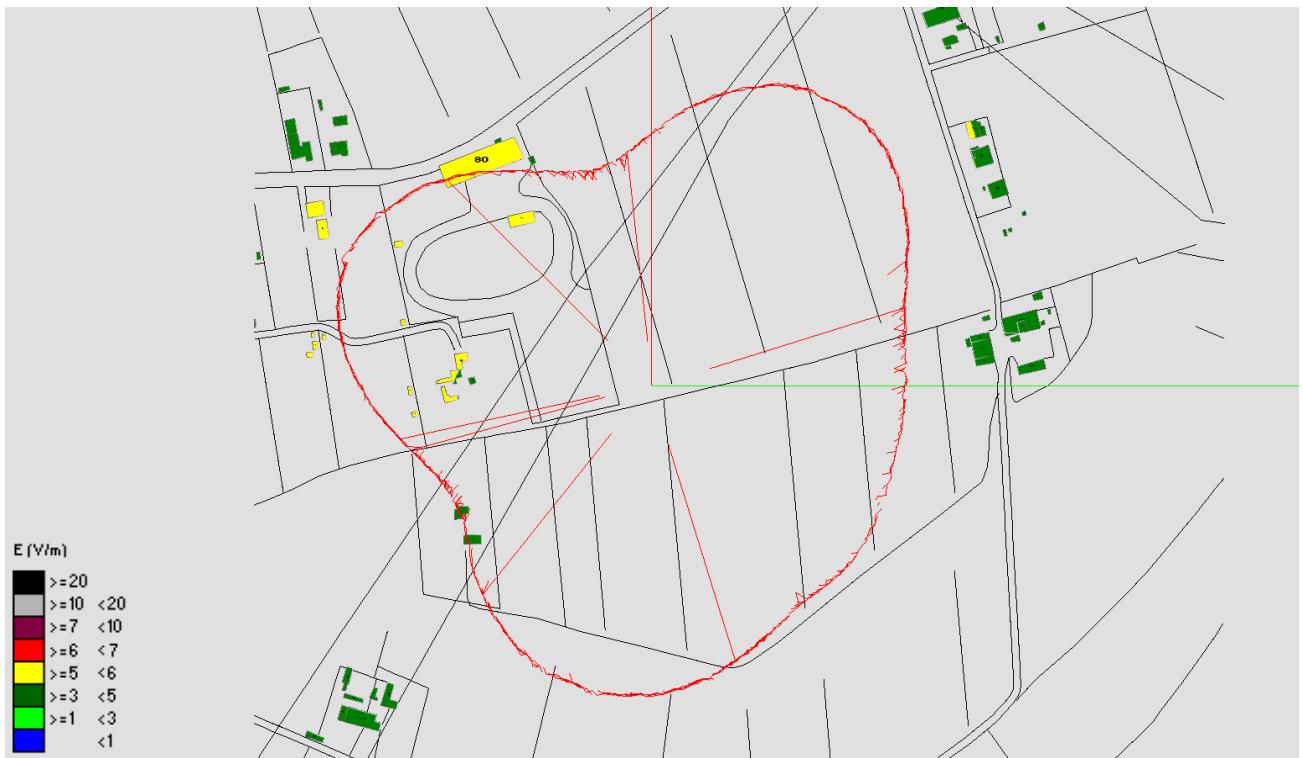
Fig. 28 Impatto elettromagnetico - Zona Area Comunale Via dei Tavi - Vista dall'alto
