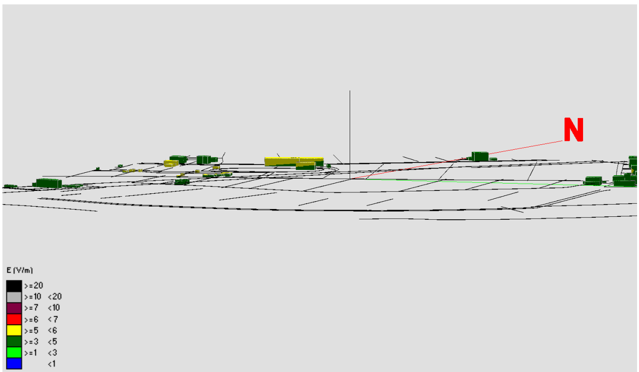
Fig. 30 Impatto elettromagnetico - Zona Area Comunale Via dei Tavi - Vista Laterale 2
