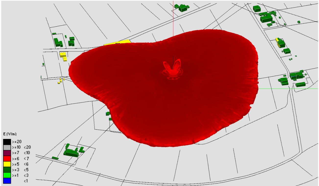
Fig. 27 Impatto elettromagnetico - Zona Area Comunale Via dei Tavi - 0°/Nord
